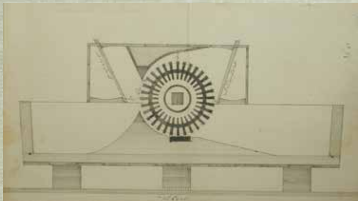
Constructietekening van een maalbak of "Hollander" door Dirk Jb de Vries op papier met watermerk van C & J HONIG [Stichting Archief Honig(h)]
