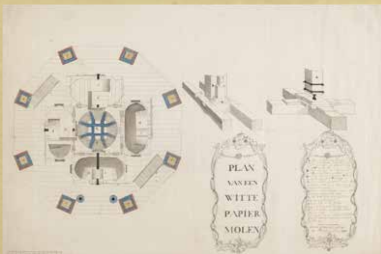
Bouwtekening grondplan witpapiermolen met vier maalbakken rond het spil door Jacob Cornelisz. Breet, 25 januari 1793. [Zaanlandia Illustratienummer. 845; GAZ 52.01195] NB: Deze tekening, behorende tot de reeks 'Plan van een witte papiermolen' was geruime tijd onvindbaar.
