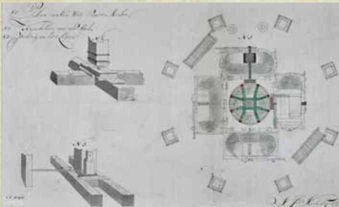
Bouwtekening voor een witte papiermolen, J.J.Kool, 6 December 1793 [Zaanlandia Illustrata nr. 848; GAZ 52.00042]
