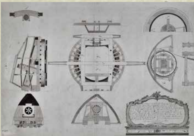
Bouwtekening van een molenkap van een papiermolen, J.J.Kool, 1793 [Zaanlandia Illustrata nr. 848; GAZ 52.00047]
