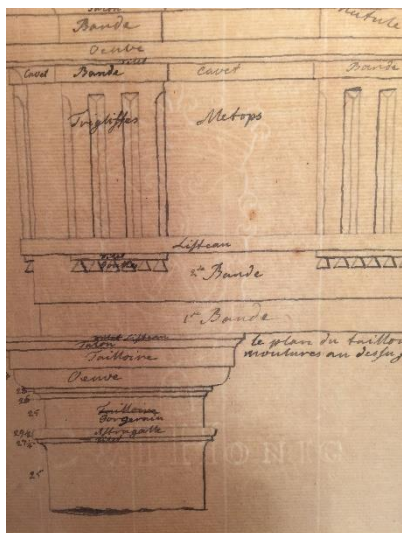
Een van de Zweedse architectuurtekeningen op papier van C & J HONIG
