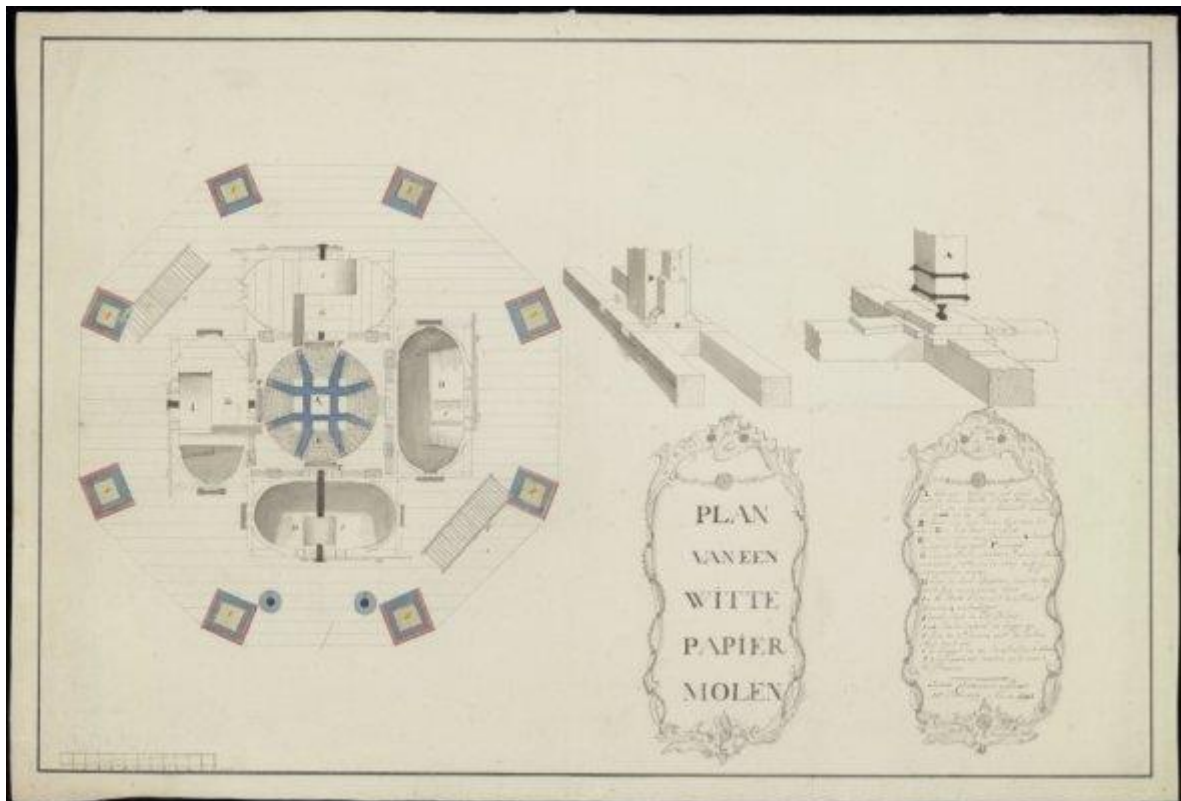
[GAZ 52.01195] Plan van een witte papiermolen door J.Cz. Breet. Lijntekening in gewassen inkt en aquarel.
