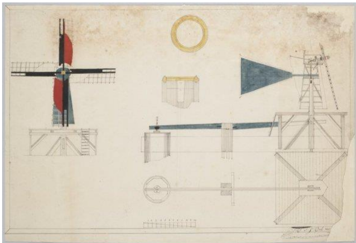
[GAZ 52.01194] Plan voor een petmolen door J.J. Kool.
